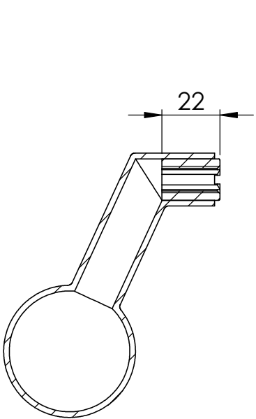
SCHNITT A-A
