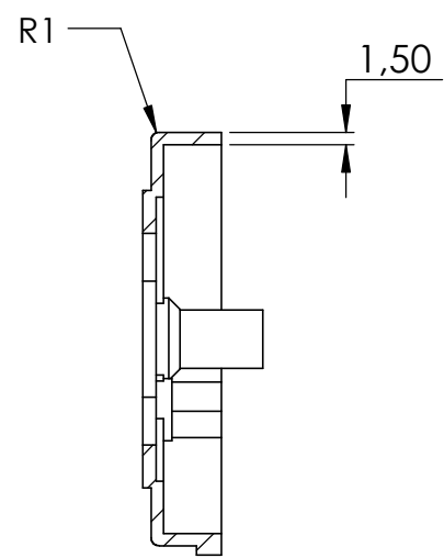
SCHNITT B-B
