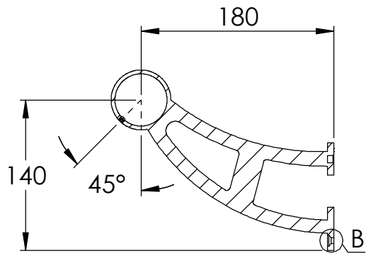
SCHNITT A-A
