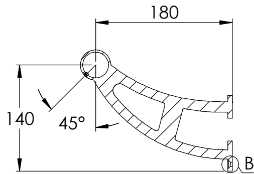
SCHNITT A-A
