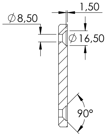
SCHNITT A-A
