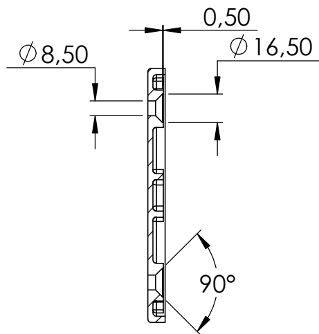
SCHNITT A-A
