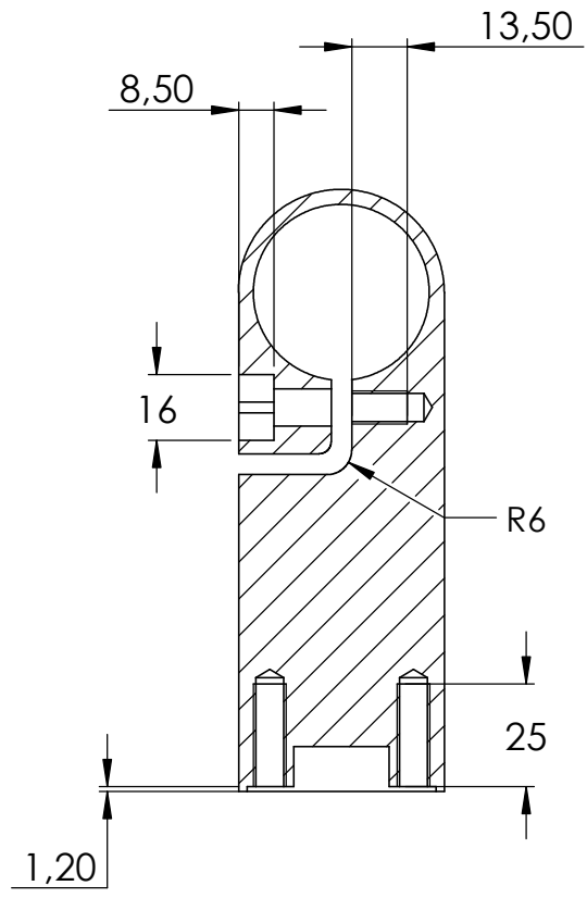
SCHNITT A-A
