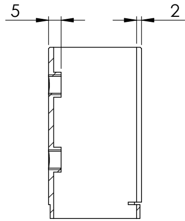
SCHNITT C-C
