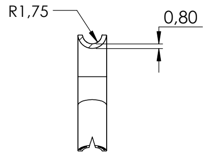
SCHNITT A-A
