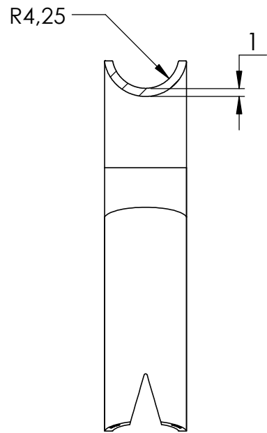
SCHNITT A-A
