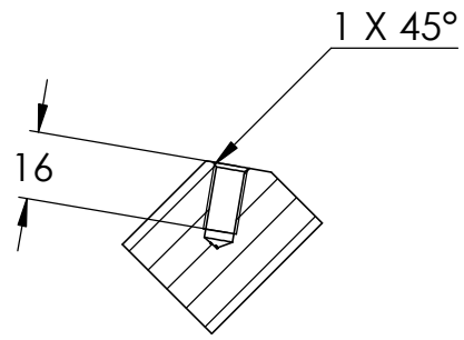
SCHNITT A-A
