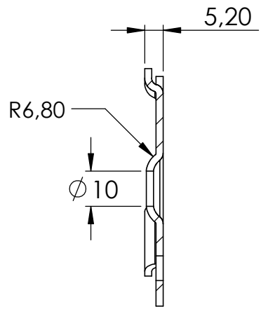
SCHNITT A-A
