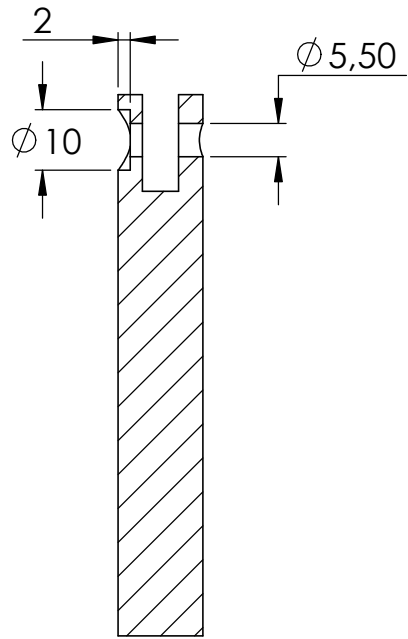
SCHNITT C-C
