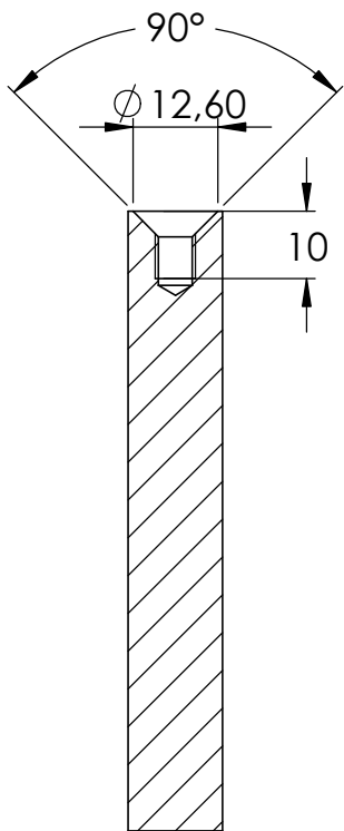
SCHNITT C-C
