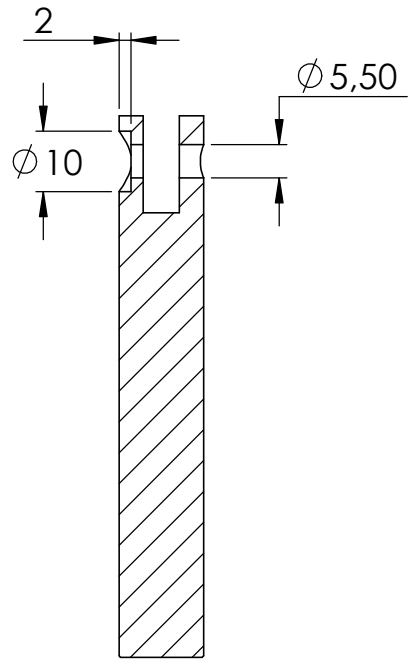
SCHNITT D-D
