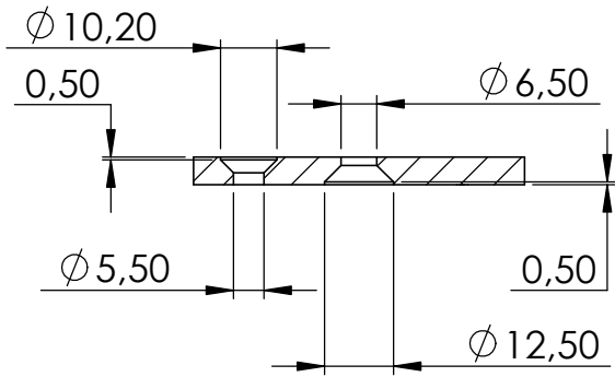
SCHNITT A-A
