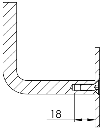
SCHNITT A-A
