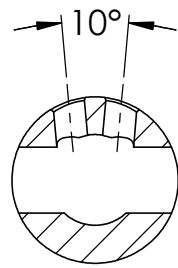
SCHNITT C-C
